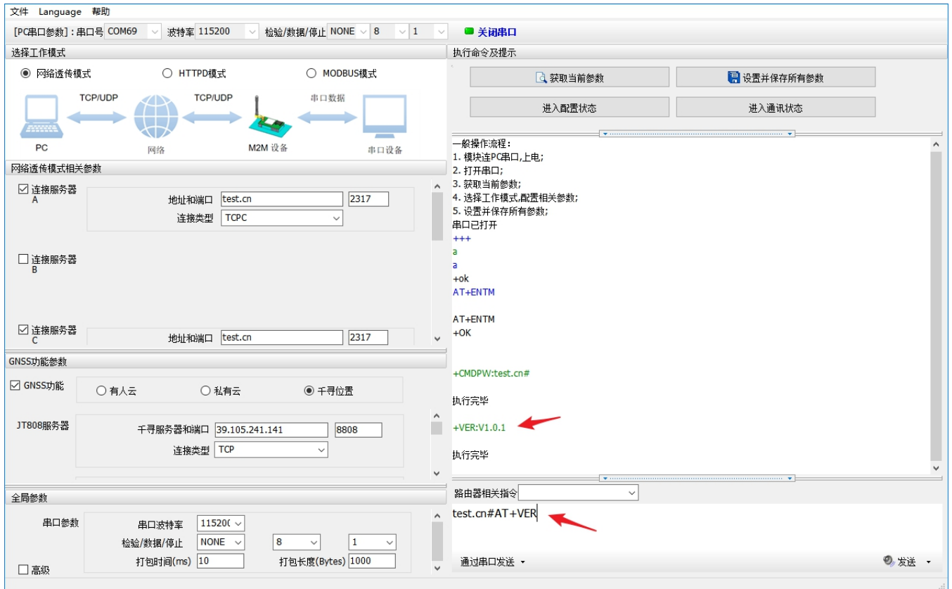
图 112 设置软件示意图
