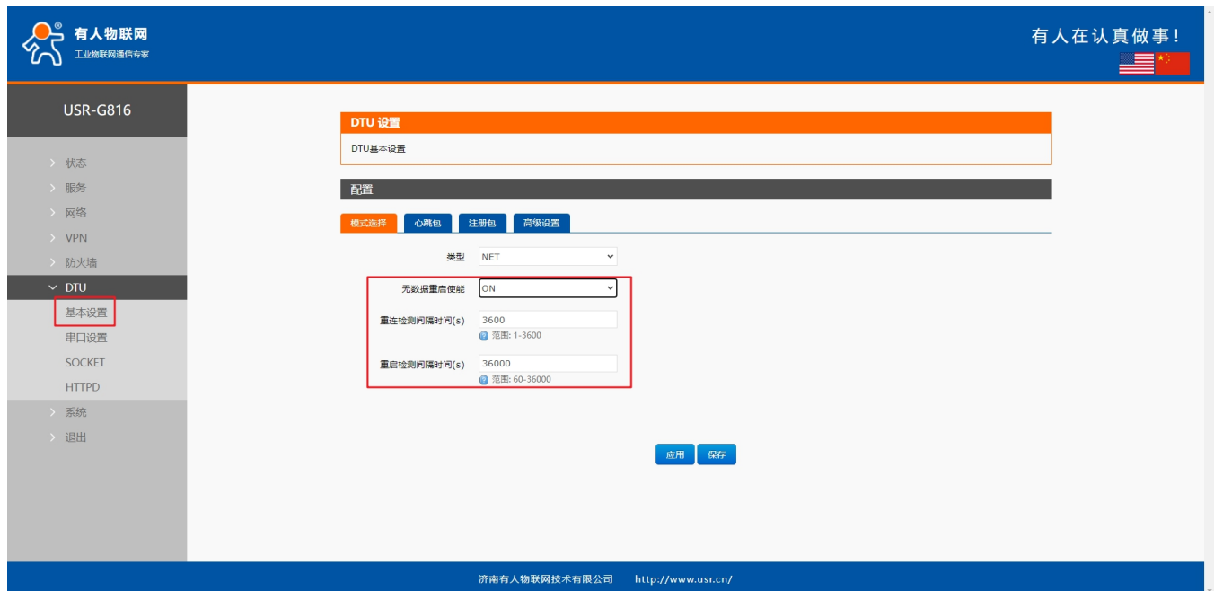
图 102 无数据重连/重启配置界面
