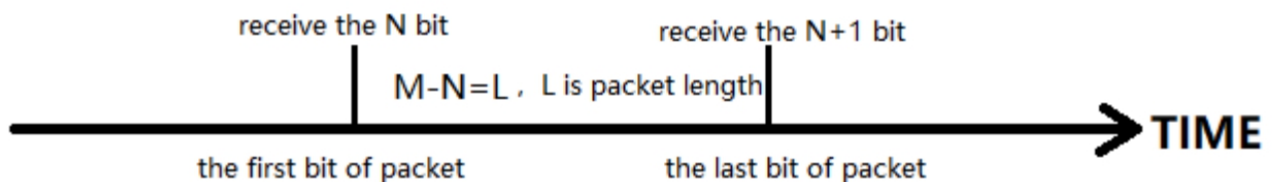
图 105 长度触发模式
