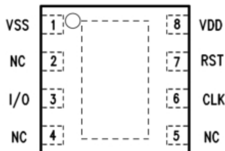
图 23 C2x2eSIM 芯片管脚示意 (TOP VIEW)
