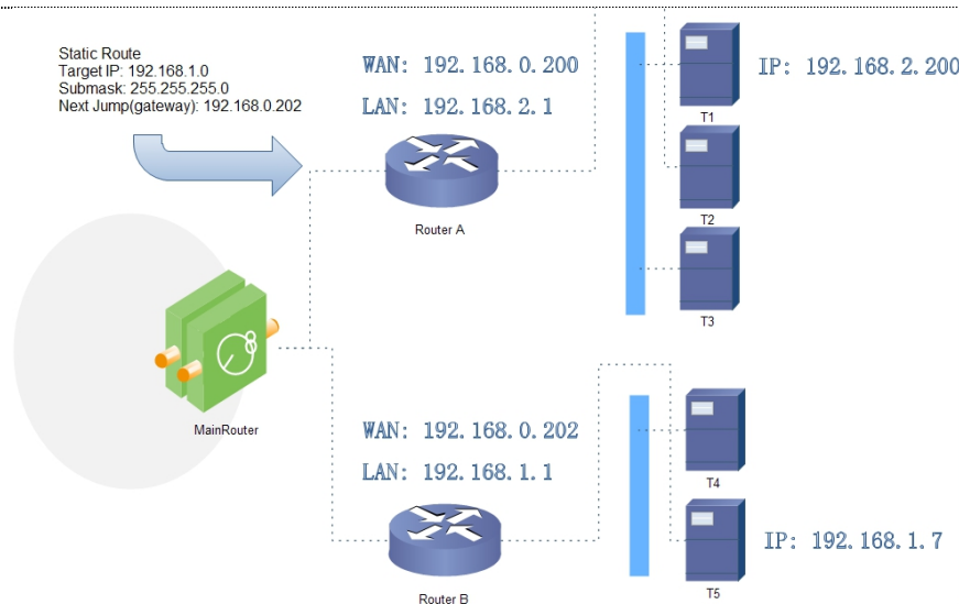
图 34 静态路由表实例图
