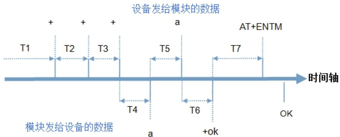
图 110 切换指令模式时序
